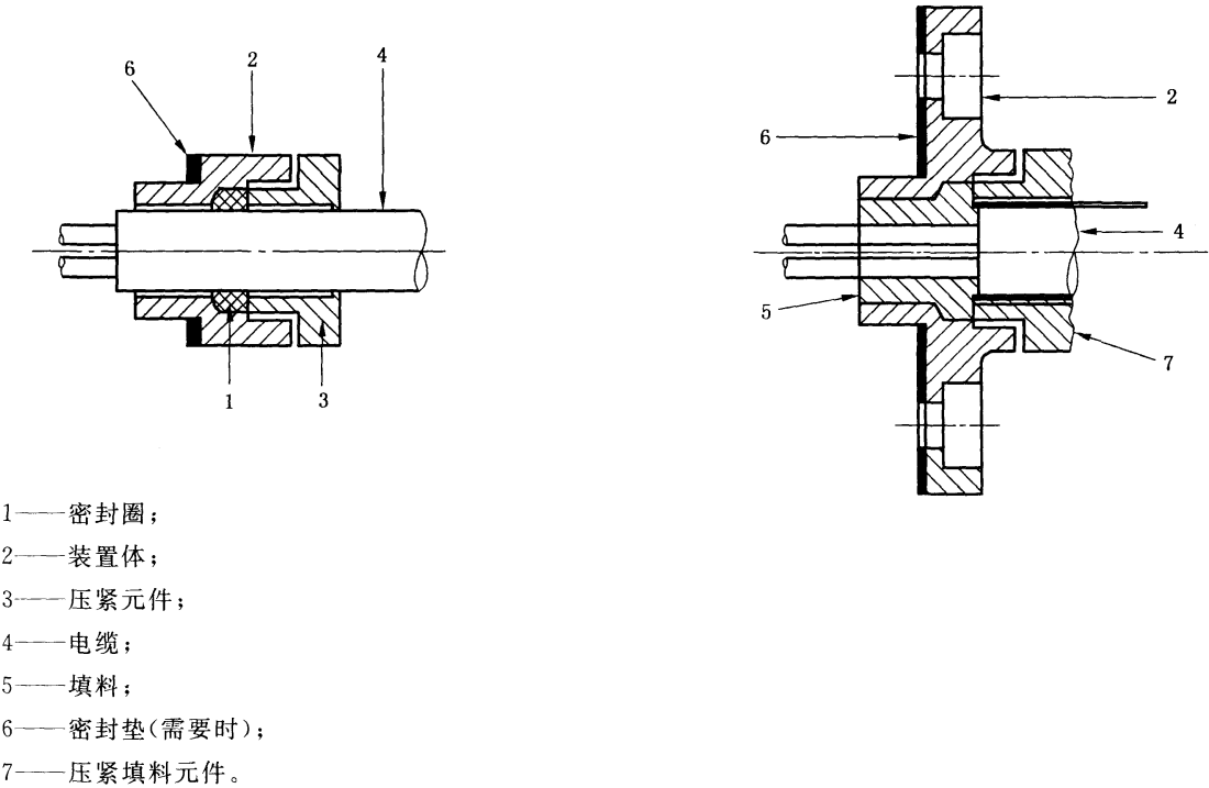
图 A.1 电缆引入装置结构示意图
