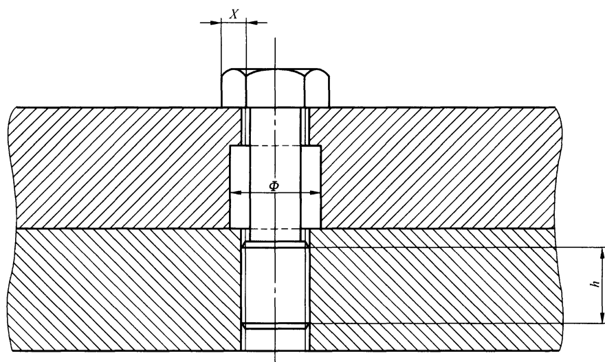
图 1 螺纹紧固件的公差和间隙
