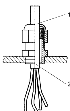
a) 电缆引入装置
