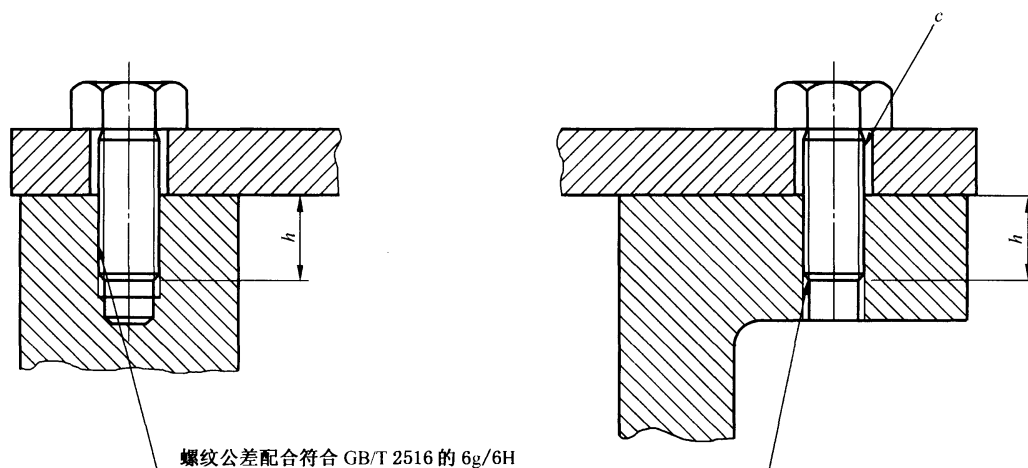
图 1 螺纹紧固件的公差和间隙
