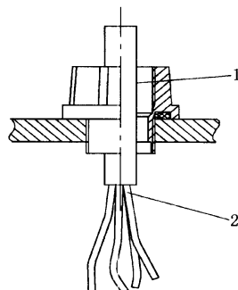
b) 导管引入方式
