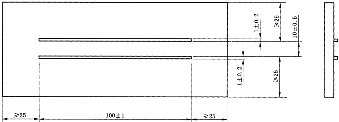
图5 涂导电漆电极的试件
